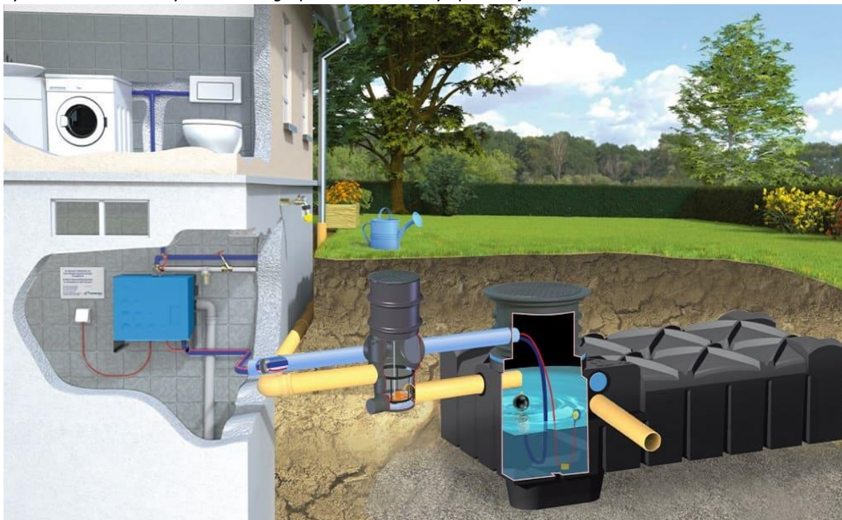
Rysunek 61. Schemat systemu do zagospodarowania wody opadowej.
